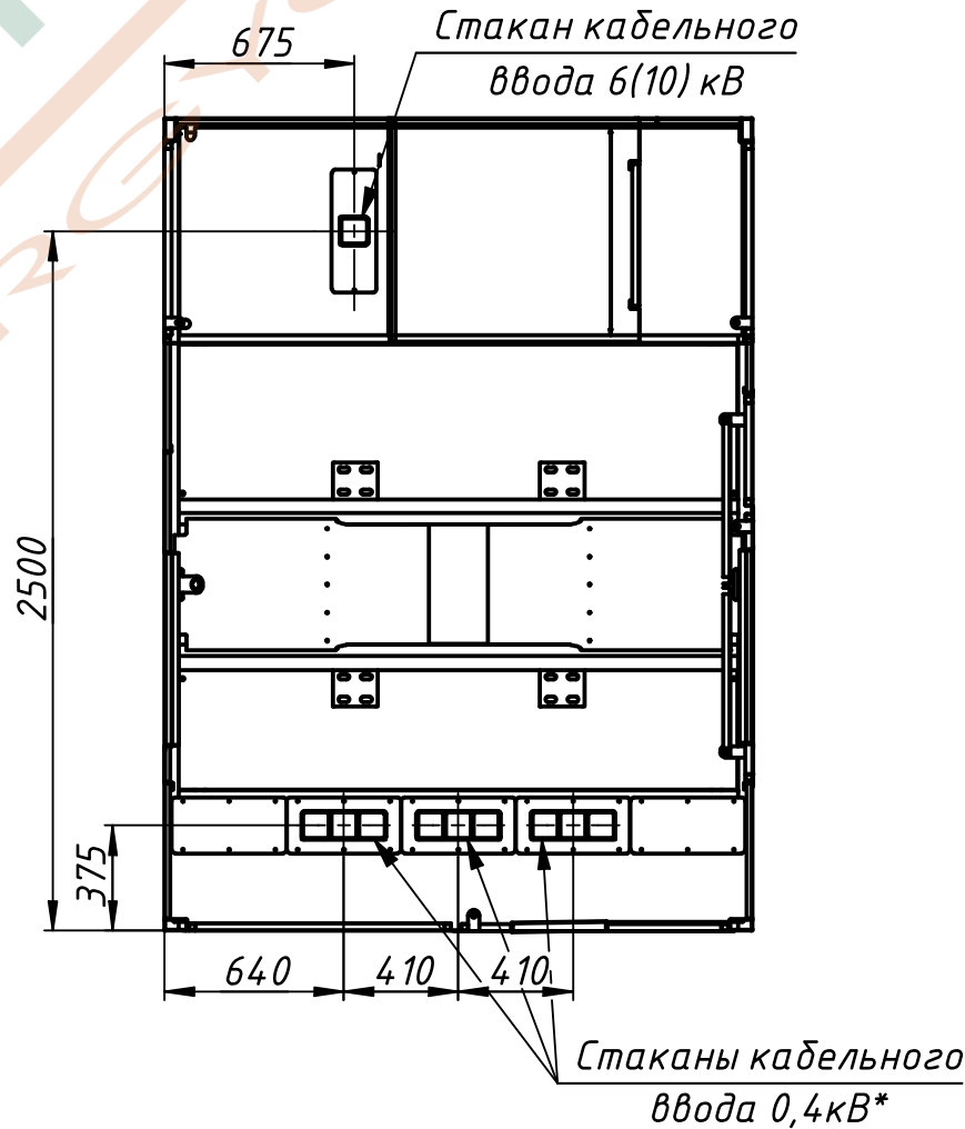
Б-Б План основания
